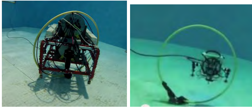
Figure 20 – Test du cerceau pour les drones sous-marins Aquatis V2 (à gauche) et Ryujin (à droite).
