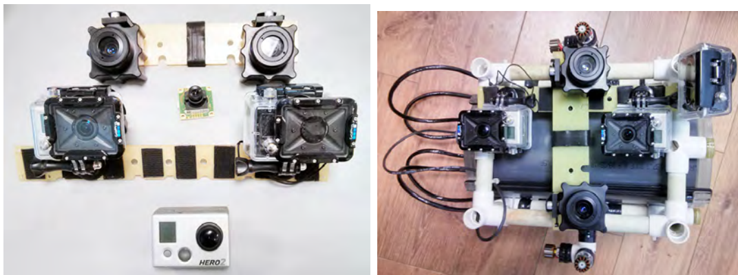
Figure 26 – Bancs stéréoscopiques synchronisés développés et testés lors de la mission terrain (à gauche) et leur intégration sur le drone Ryujin (à droite).
