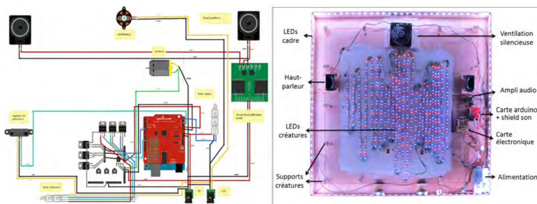
Figure 13 – Schéma électrique et électronique et réalisation
