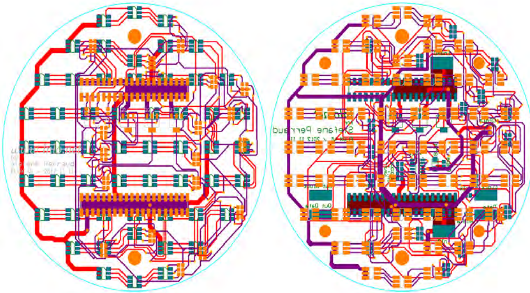
Figure 8 – Circuit imprimé recto et verso de Flux. Design par Laurent Brun.
