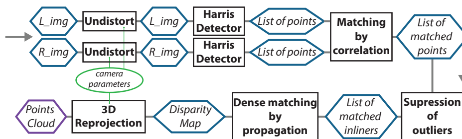
Figure 29 – La chaîne de reconstruction 3D.
