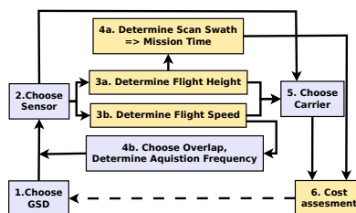
Figure 31 – Extrait de la méthodologie de la RTE pour guider aux choix du porteur, de la charge utile et des paramètres d'acquisition.
