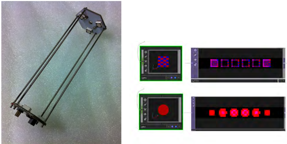
Figure 4 – Module de LEDs, 2 pixels, 6 LEDs, avec connecteurs pour le relier à d'autres (à gauche) - Deux exemples de décomposition en plans d'objets 3D : un cube vide et une sphère pleine (à droite).
