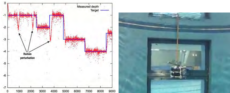
Figure 21 – Asservissement en profondeur : à gauche la consigne en profondeur (courbe bleue) et la profondeur réelle du sous-marin (courbe rouge) et à droite Ryujin en train d’être perturbé.
